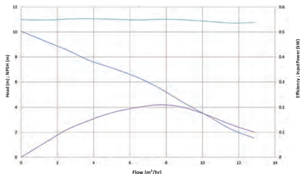
Aquamite 100
